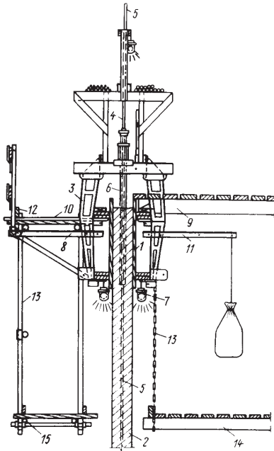
Рисунок 7. Схема крепления уравнивающей консоли (1 — щит опалубки; 2 — железобетонная стена; 3 — домкратная рама; 4 — гидродомкрат; 5 — домкратный стержень; 6 — защитная трубка; 7 — осветительное оборудование; 8 — консоль для опирания верхней наружной рабочей площадки; 9 — верхняя внутренняя рабочая площадка; 10 — верхняя наружная рабочая площадка; 11 — уравнивающая консоль; 12 — перила ограждения; 13 — вертикальные тяги крепления нижней рабочей площадки; 14 — нижняя внутренняя рабочая площадка; 14 — нижняя наружная рабочая площадка)
