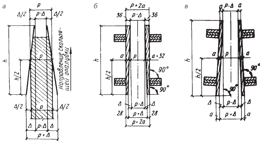
Рисунок 2. Схема устройства конусности опалубки (а – принципиальная схема устройства конусности опалубки; б – схема устройства конусности опалубки за счет конструкции щитов; в – схема устройства конусности опалубки за счет способа крепления щитов при монтаже)
