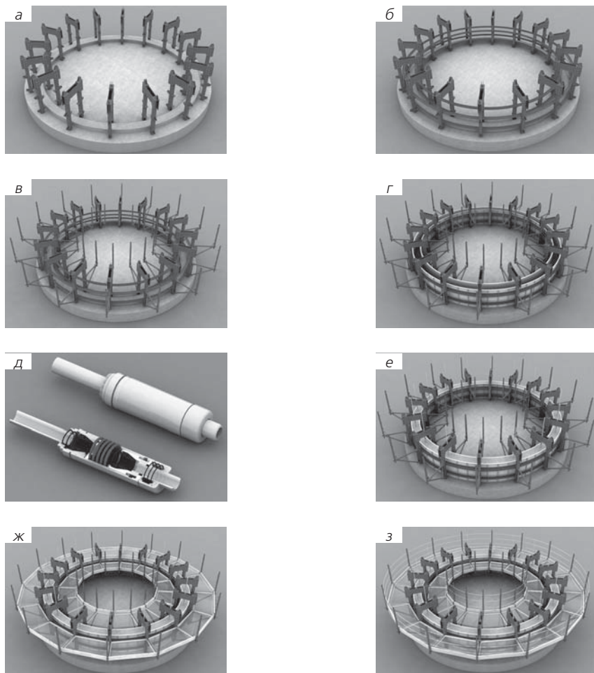
Рисунок 4. Технологическая последовательность монтажа скользящей опалубки (а – установка домкратных рам; б – фиксация элементов обрешетки (кружал); в – то же консолей для опирания верхних наружной и внутренней рабочих площадок; г – монтаж щитов скользящей опалубки; д – схема гидродомкрата; е – установка гидродомкрата на домкратную раму; ж – то же верхних наружных и внутренних рабочих площадок; з – то же перил ограждения)
