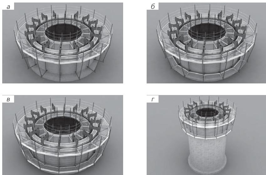
Рисунок 8. Технологическая последовательность монтажа нижних внутренней и наружной рабочих площадок (а – фиксация вертикальных тяг для монтажа нижних рабочих площадок; б – то же настила нижних рабочих площадок; в – установка перил ограждения нижних рабочих площадок)
