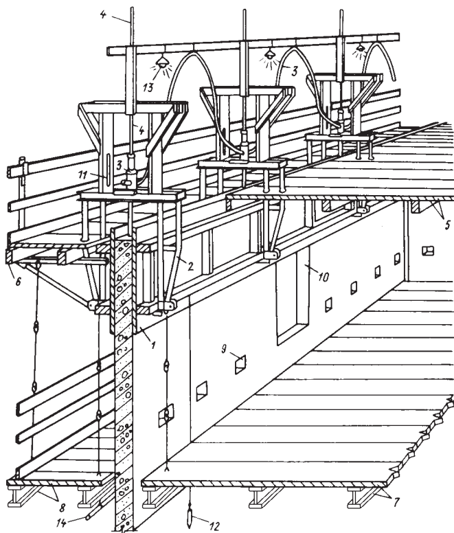
Рисунок 1. Общий вид скользящей опалубки (1 — щит опалубки; 2 — домкратная рама; 3 — гидродомкрат; 4 — домкратные стержни; 5 — верхняя внутренняя рабочая площадка; 6 — верхняя наружная рабочая площадка; 7 — нижняя внутренняя рабочая площадка; 8 — нижняя наружная рабочая площадка; 9 — отверстия для опирания перекрытия; 10 — дверной (оконный) проем; 11 — оборудование для контроля горизонтальности скользящей опалубки; 12 — оборудование для контроля вертикальности сооружения; 13 — электрическое оборудование; 14 — система водоснабжения)
