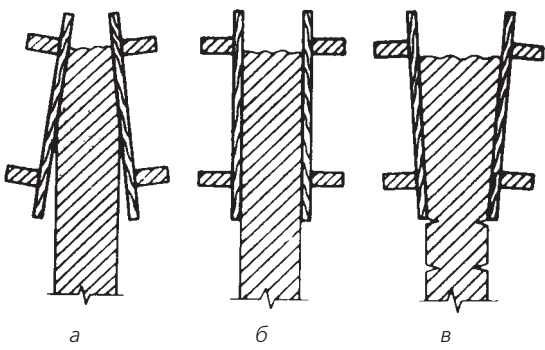
Рисунок 3. Схема формирования конусности скользящей опалубки (а – щиты установлены правильно (конусность опалубки по направлению скольжения); б – щиты установлены неправильно (не имеют наклона); в – щиты установлены неправильно (конусность опалубки против направления скольжения))
