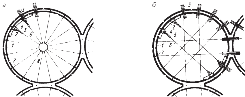
Рисунок 5. Схемы расположения горизонтальных тяг круглой скользящей опалубки (а – радиальное расположение горизонтальных тяг; б – парное расположение горизонтальных тяг). 1 – стенка; 2 – ребро; 3 – домкратная рама; 4 – скоба для крепления горизонтальной тяги к щиту скользящей опалубки; 5 – муфта для натягивания горизонтальной тяги; 6 – горизонтальная тяга; 7 – домкратный стержень; 8 – центровочный диск (кольцо) для крепления горизонтальных тяг)
