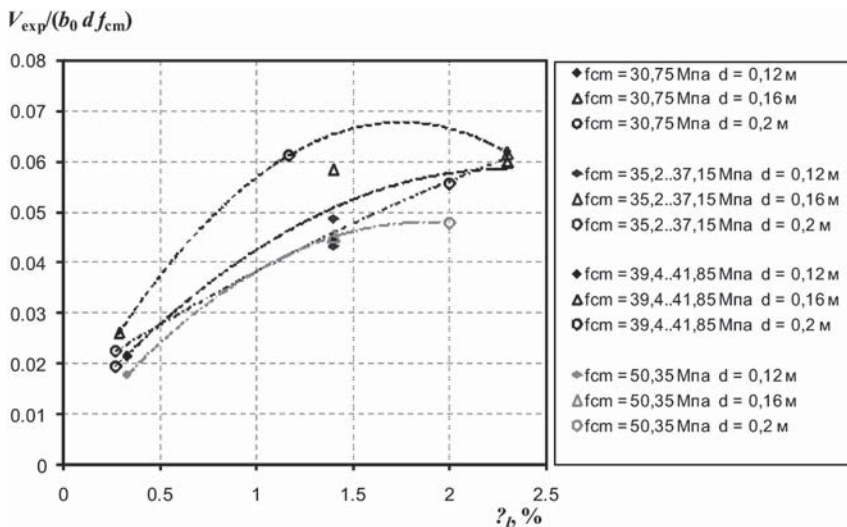
Рисунок 9. График изменения относительной перерезывающей силы при различной прочности бетона на осевое сжатие
