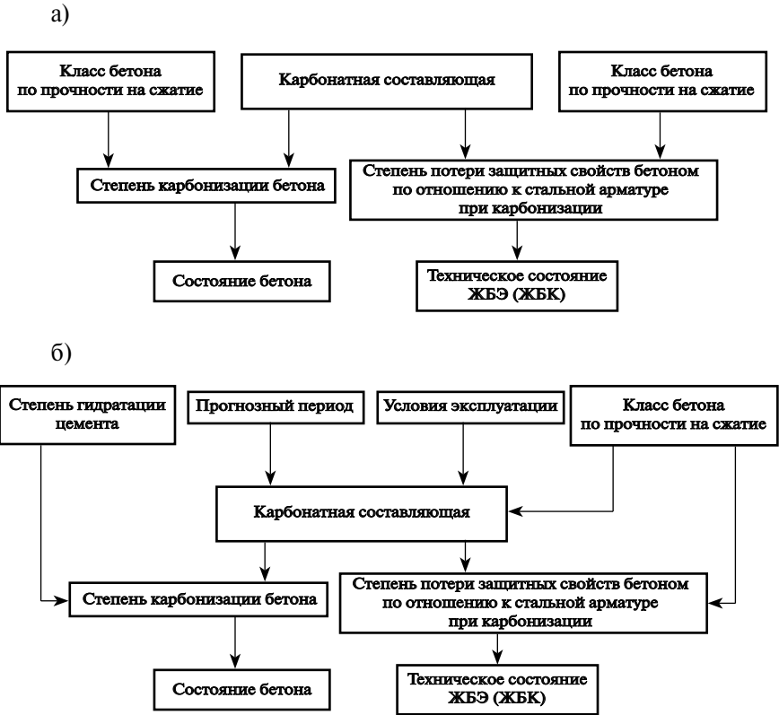
Рисунок 1. Структурная схема комплексного метода оценки и прогнозирования технического состояния ЖБЭ (ЖБК), эксплуатирующихся в различных атмосферных условиях, с учетом карбонизации бетона:
