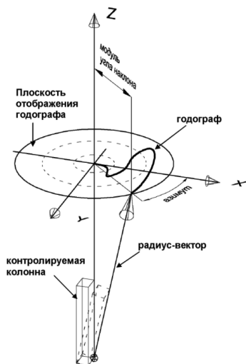
Рисунок 6. Схема отображения данных угловых отклонений колонн здания
